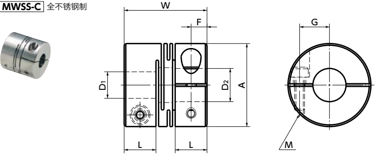
MWSS-C 全不锈钢制
