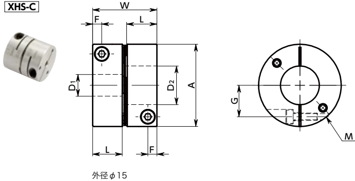
XHS-C
