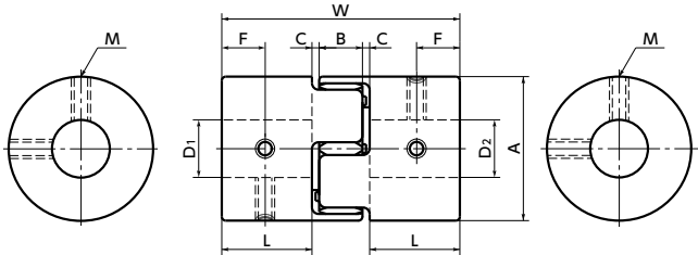
外径 \phi 40
