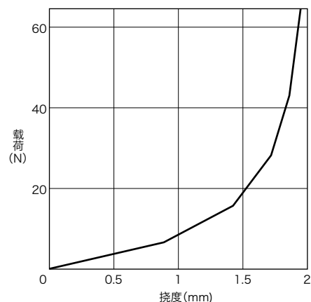
· 以不等间距开槽，以近似2次曲线表示弹簧特性的Flexus。
