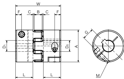
外径: \phi 55 - \phi 95
