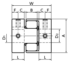
外径φ30
