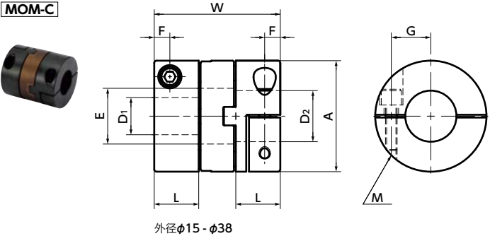
外径φ15 - φ38
