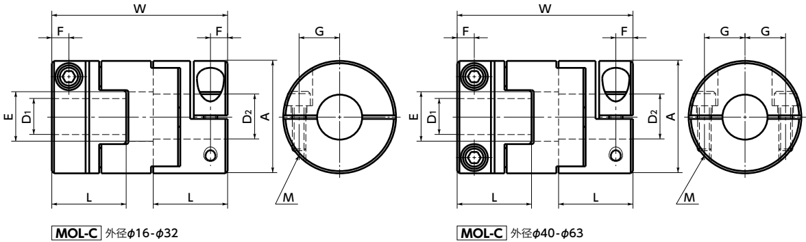
MOL-C 外径φ16-φ32
