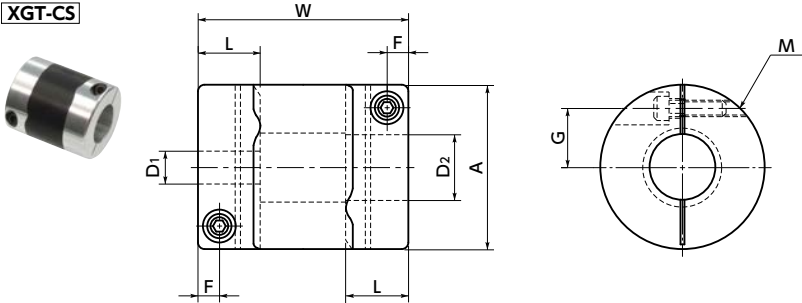
XGT-CS
