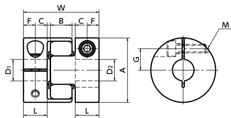
外径 \phi 14 - \phi 30
