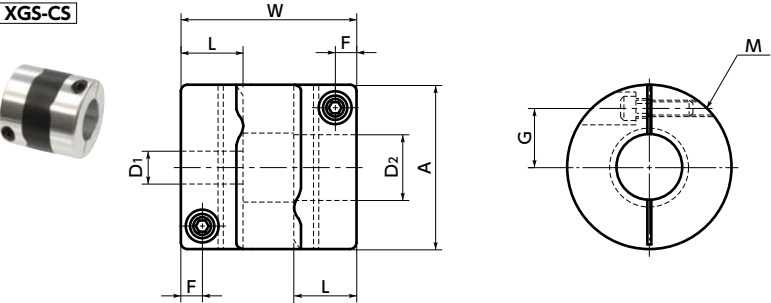
XGS-CS
