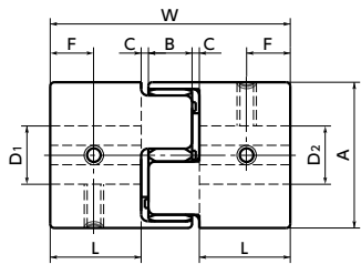
外径φ40
