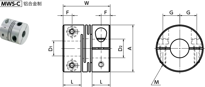
MWS-C 铝合金制
