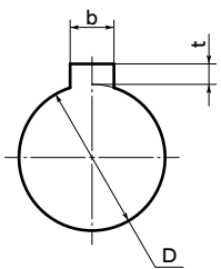
● 轴孔部详图
