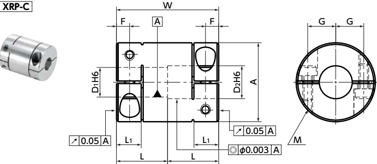
XRP-C
