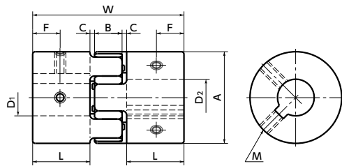
外径φ55-φ95
